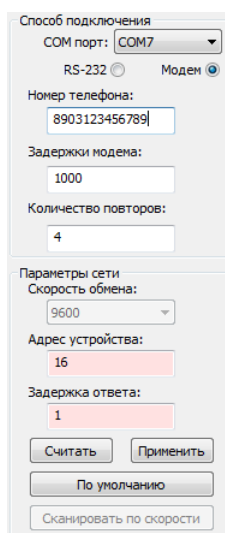
Рисунок 7.3 – Вид меню при подключении с использованием модема
