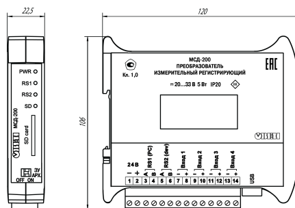
Рисунок 4.2 – Габаритные размеры
